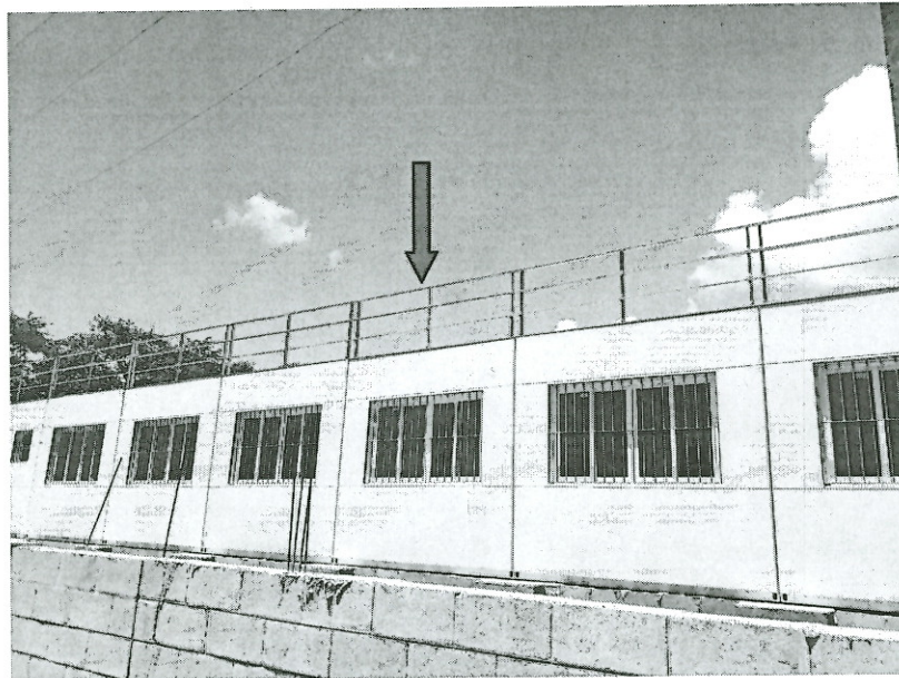
Suportes metálicos das platibandas sendo executados
